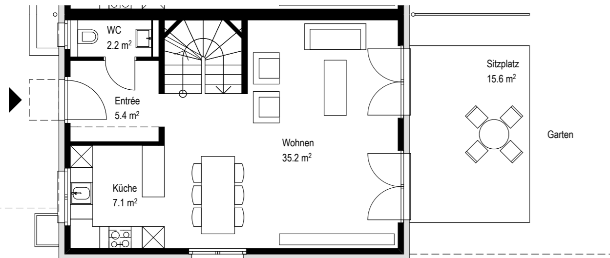
GRUNDRISS ERDGESCHOSS
