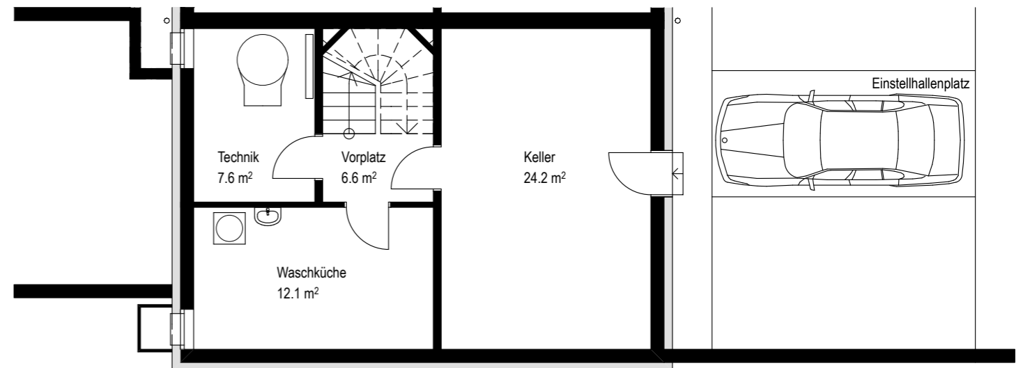
GRUNDRISS UNTERGESCHOSS
