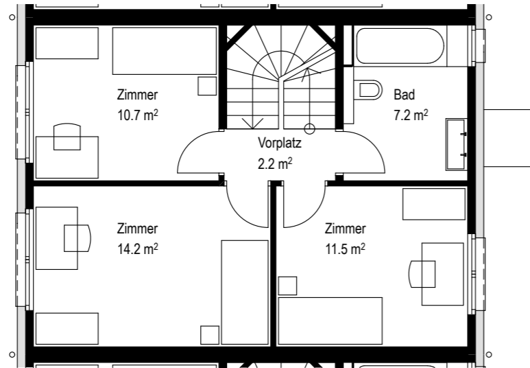
GRUNDRISS OBERGESCHOSS
