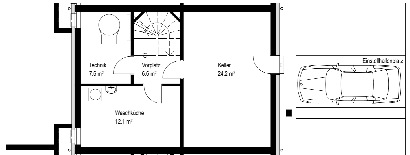
GRUNDRISS UNTERGESCHOSS
