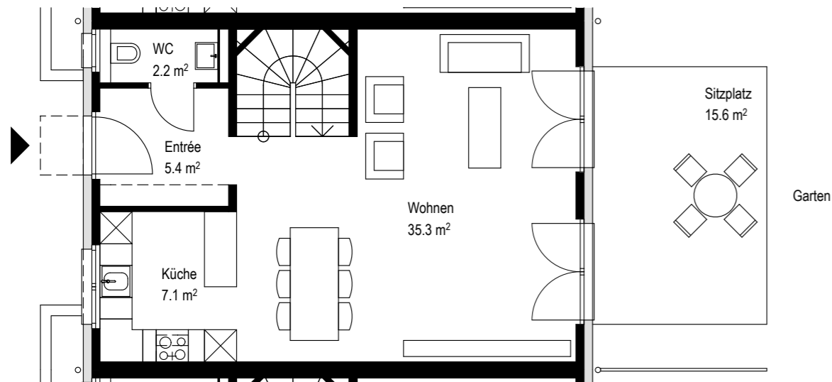
GRUNDRISS ERDGESCHOSS
