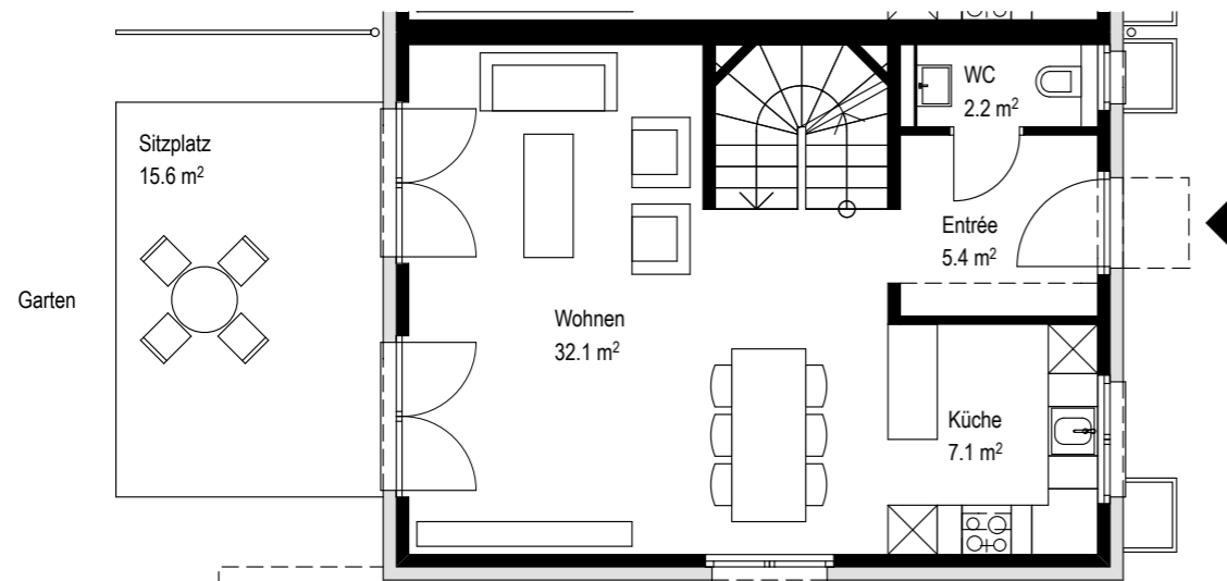
GRUNDRISS ERDGESCHOSS
