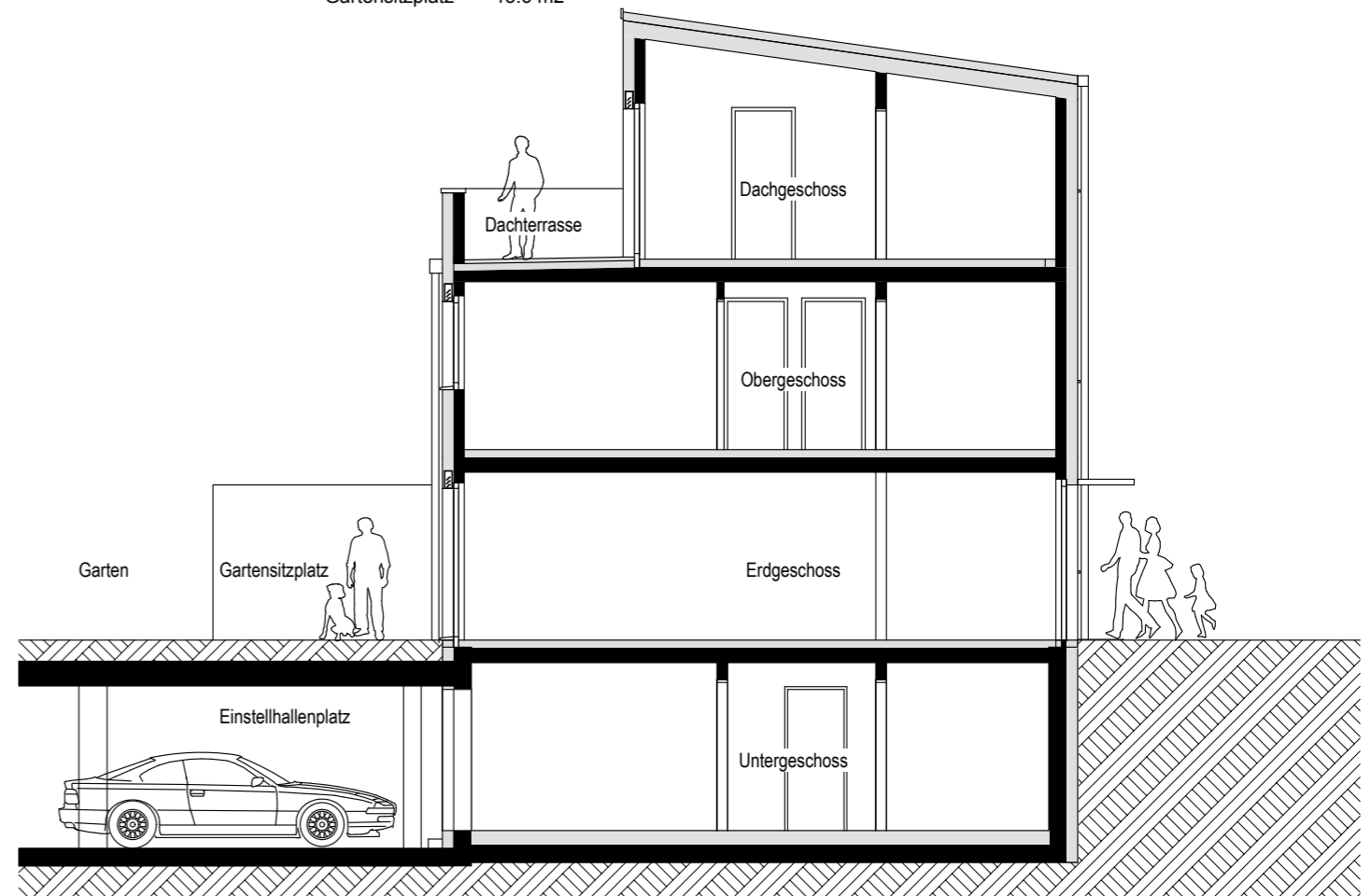
QUERSCHNITT
