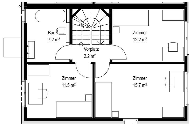
GRUNDRISS OBERGESCHOSS
