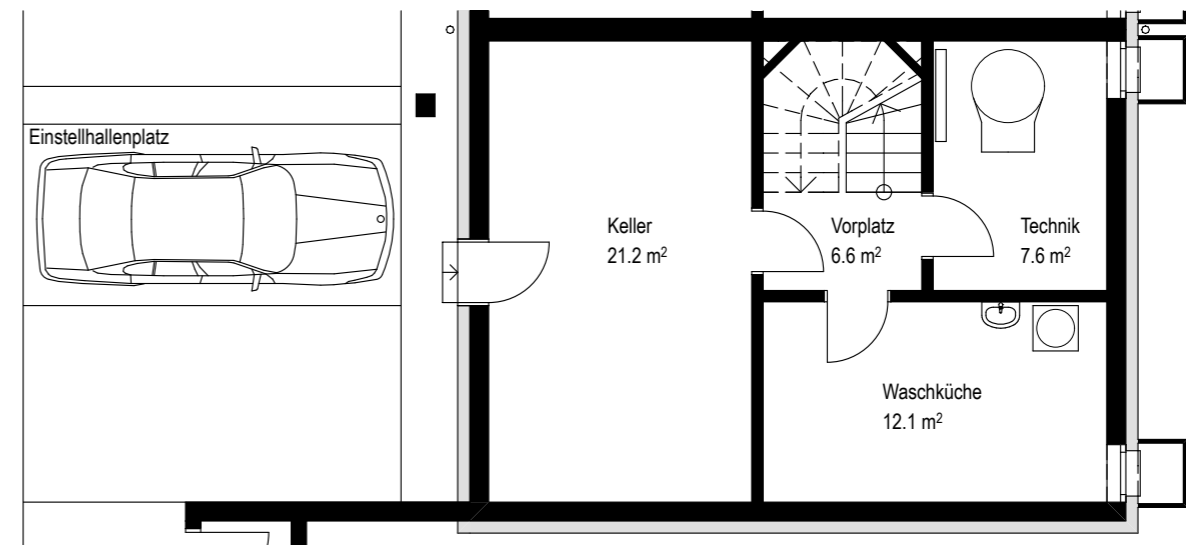
GRUNDRISS UNTERGESCHOSS
