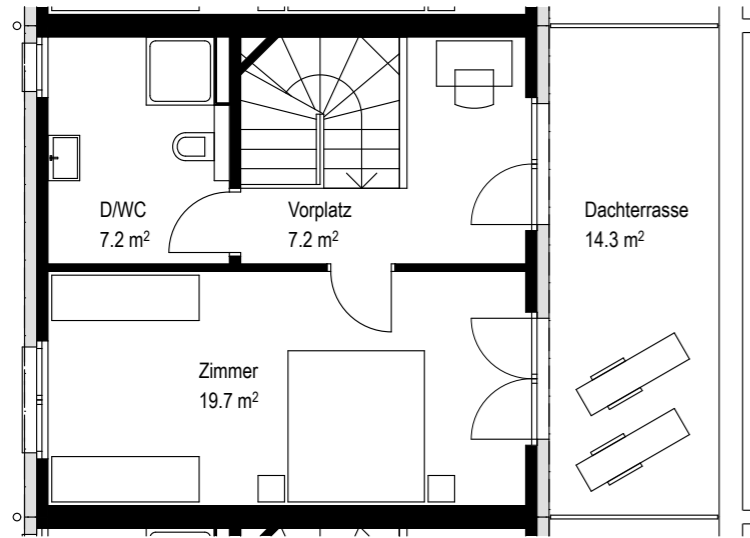
GRUNDRISS DACHGESCHOSS
