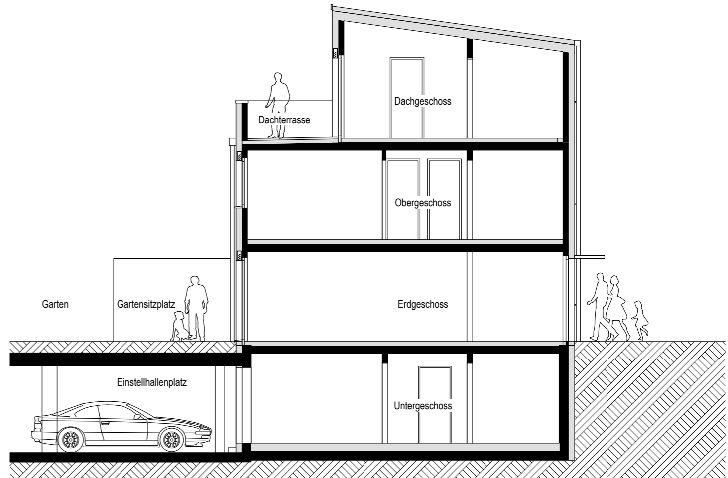
QUERSCHNITT
