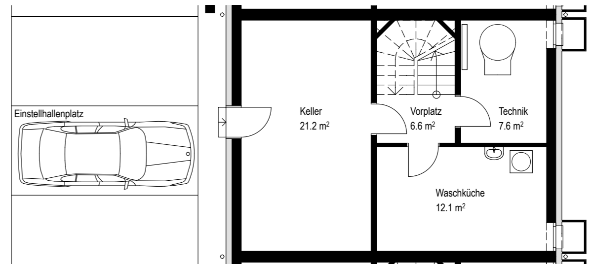
GRUNDRISS UNTERGESCHOSS
