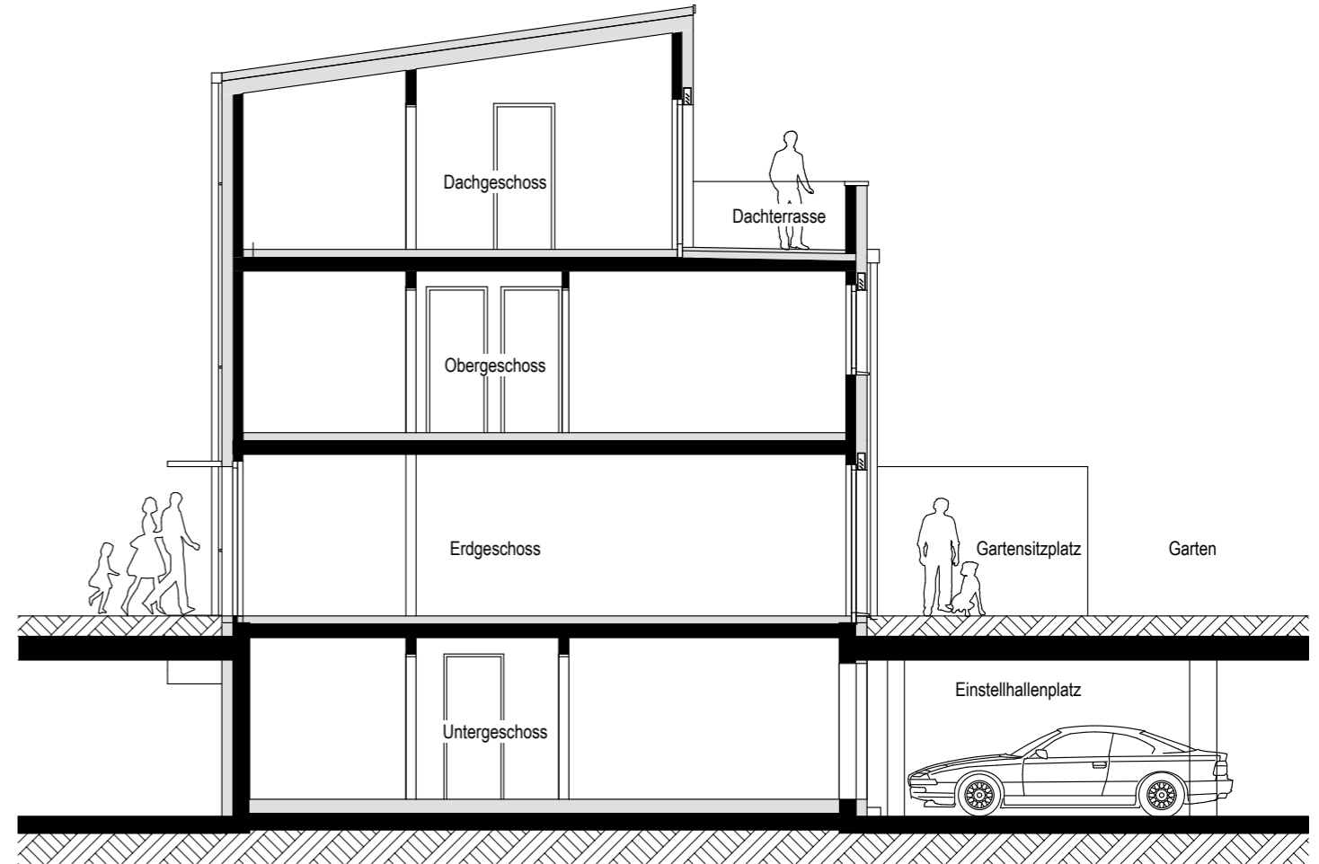
QUERSCHNITT
