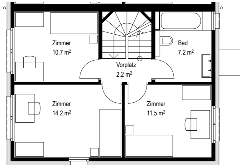
GRUNDRISS OBERGESCHOSS
